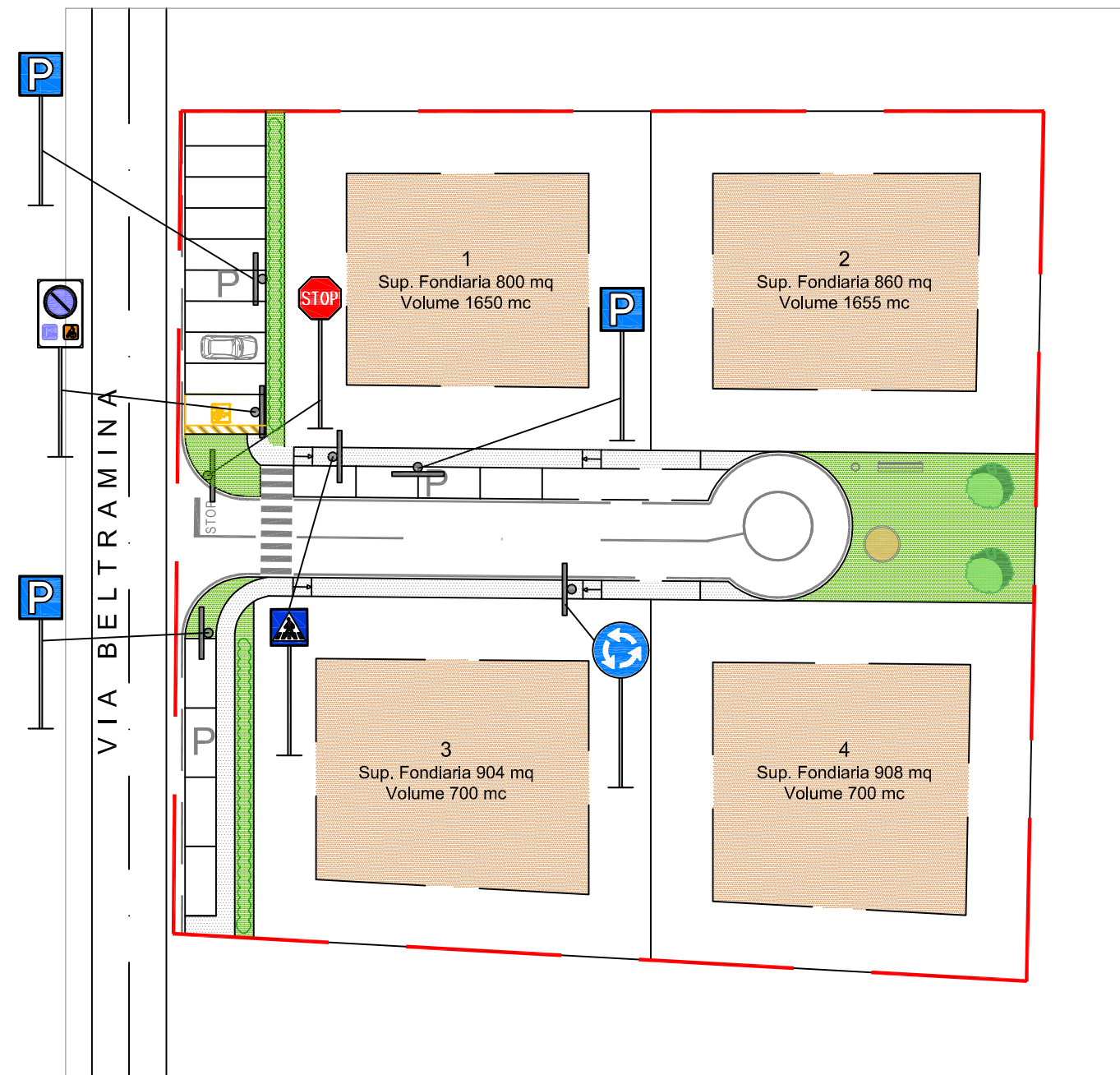
Planimetria - scala 1:500
